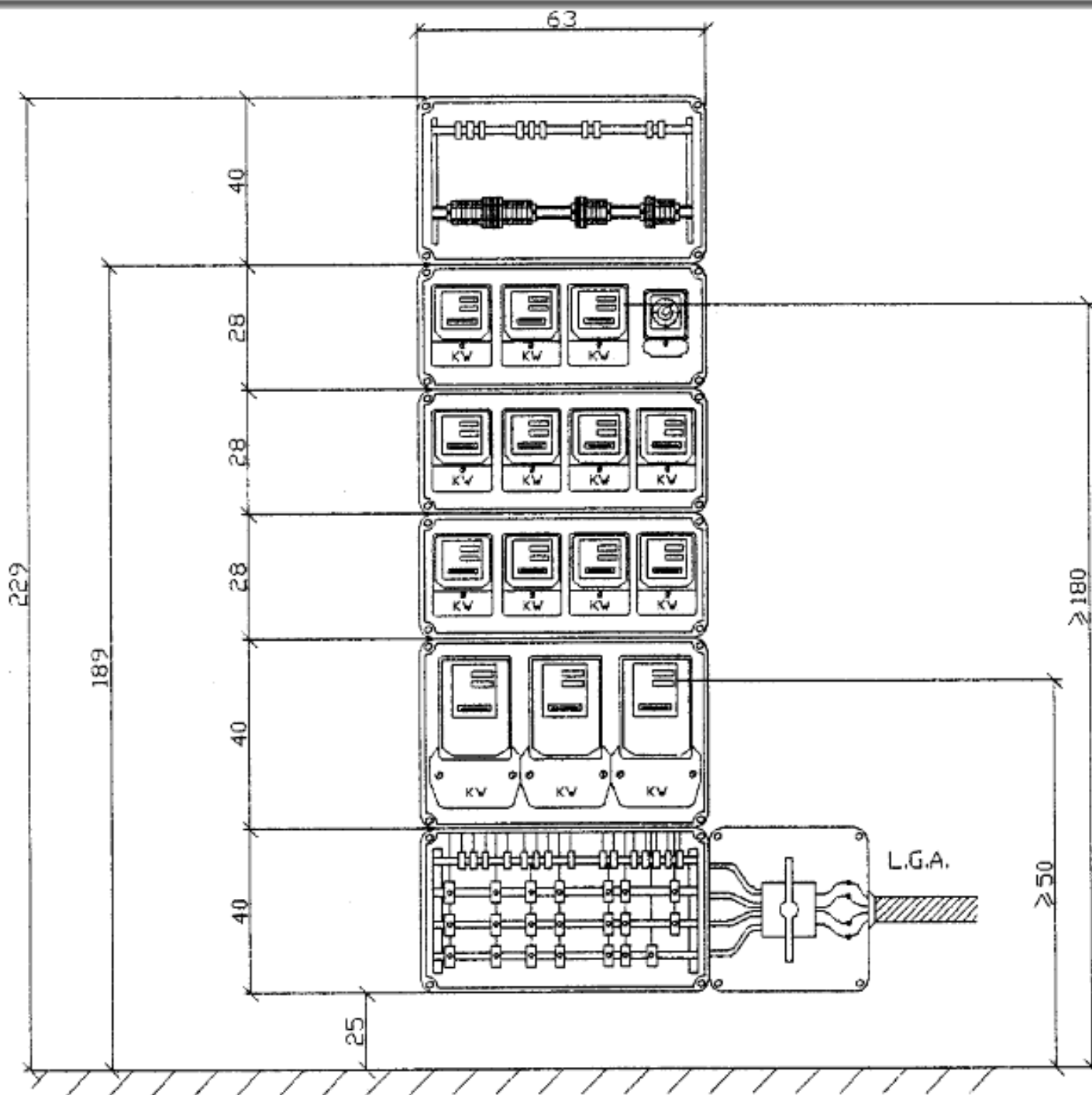
Columna de centralización de contadores
